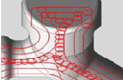
Trochoidales Fräsen mit dem Edgecam Schrappzyklus
